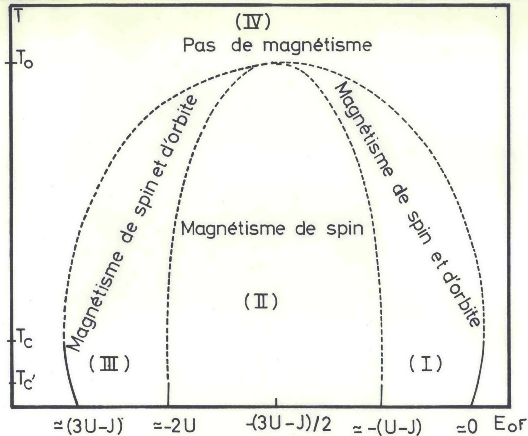
Fig-19 : Discussion en fonction de E_0F et de la température pour \frac{U}{\Delta} et \frac{J}{\Delta} donnés.
